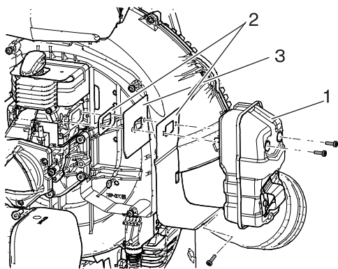
1. Silencieux
