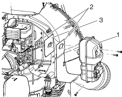
1. Silenciador 2. Junta 3. Placa de aluminio
