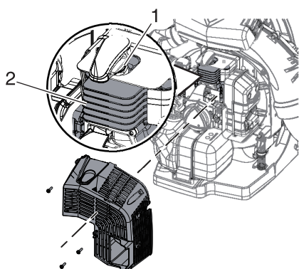
2. Aletas del cilindro
