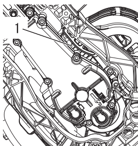
1. Ailettes de cylindre
