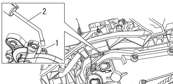
1. Raccordo di ingrassaggio 2. ingrassatore a siringa
