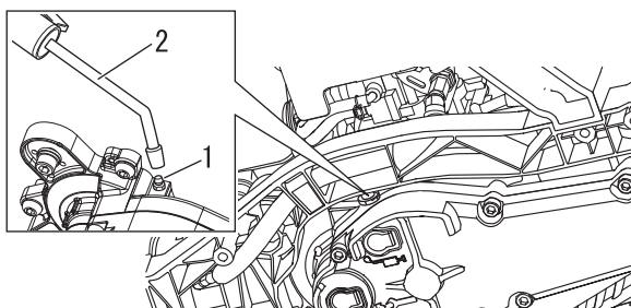
1. Orificio para grasa
