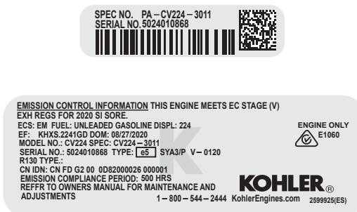
Typenschild des Kohler Motors
