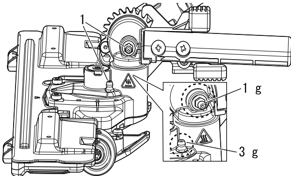
1. Schmiernippel
