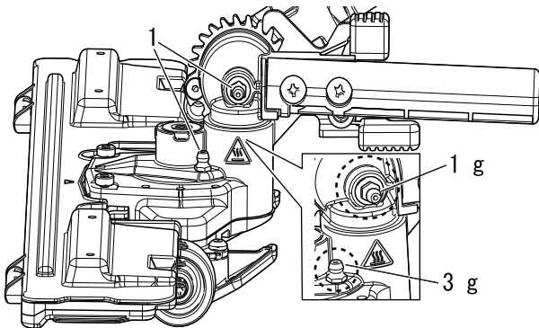
1. Graisseur
