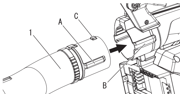
1. Rohr
