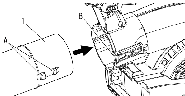
1. Blower pipe
