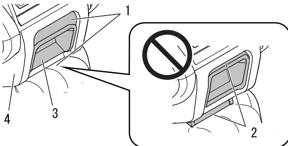
1. Eingerastet 2. Nicht eingerastet 3. Akkuverriegelung 4. Akku
