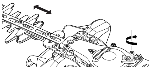
1. Bouchon fileté 2. Vis M4 d'une longueur de plus de 15 mm
