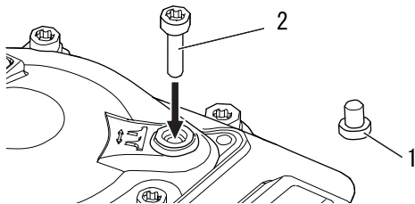
1. Verschlusschraube 2. M4-Schraube mit mehr als 15 mm Länge
