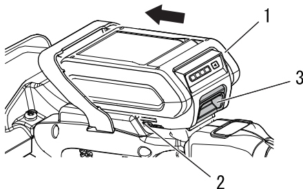
1. Akku 2. Rippe 3. Akkuverriegelung
