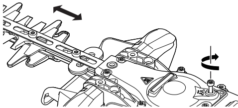
1. Verschlusschraube 2. M4-Schraube mit mehr als 15 mm Länge
