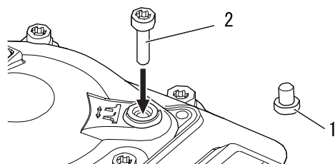
1. Bouchon fileté 2. Vis M4 d'une longueur de plus de 15 mm
