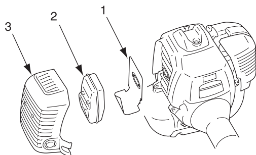
1. Ecran thermique 3. Couvercle 2. Silencieux
