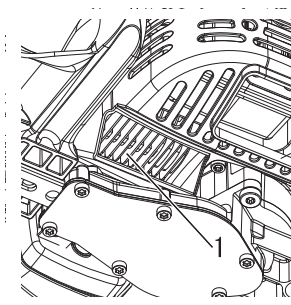
1. Zylinderrippen
