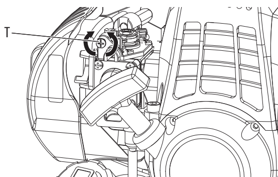
T: Leerlaufanschlagschraube
