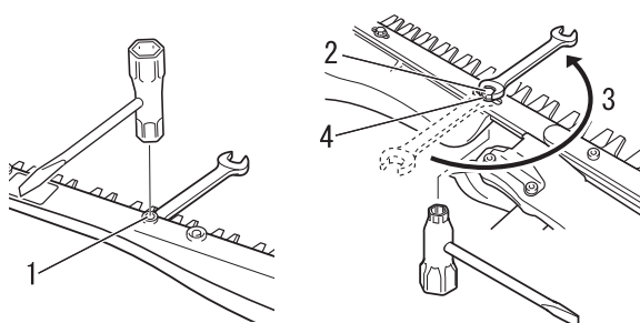
1. Contratuerca 2. Perno
