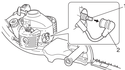
1. Zündkerze
