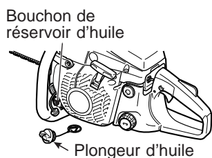
Bouchon de réservoir d'huile Plongeur d'huile
