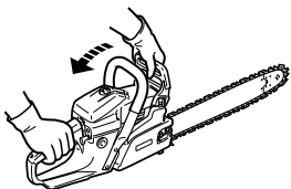
Re-armement du frein de chaîne
