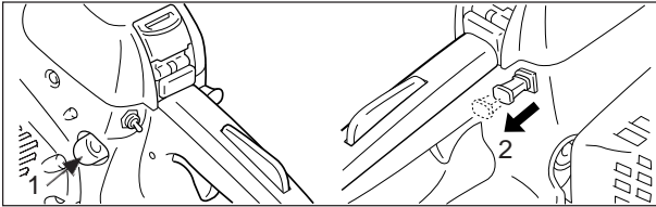
1. Primer pump 2. Choke control knob
